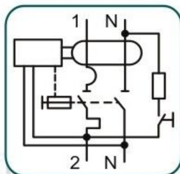
مدار الکتریکی
